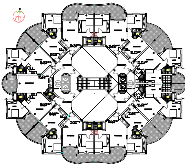
Piano tipo (11)
