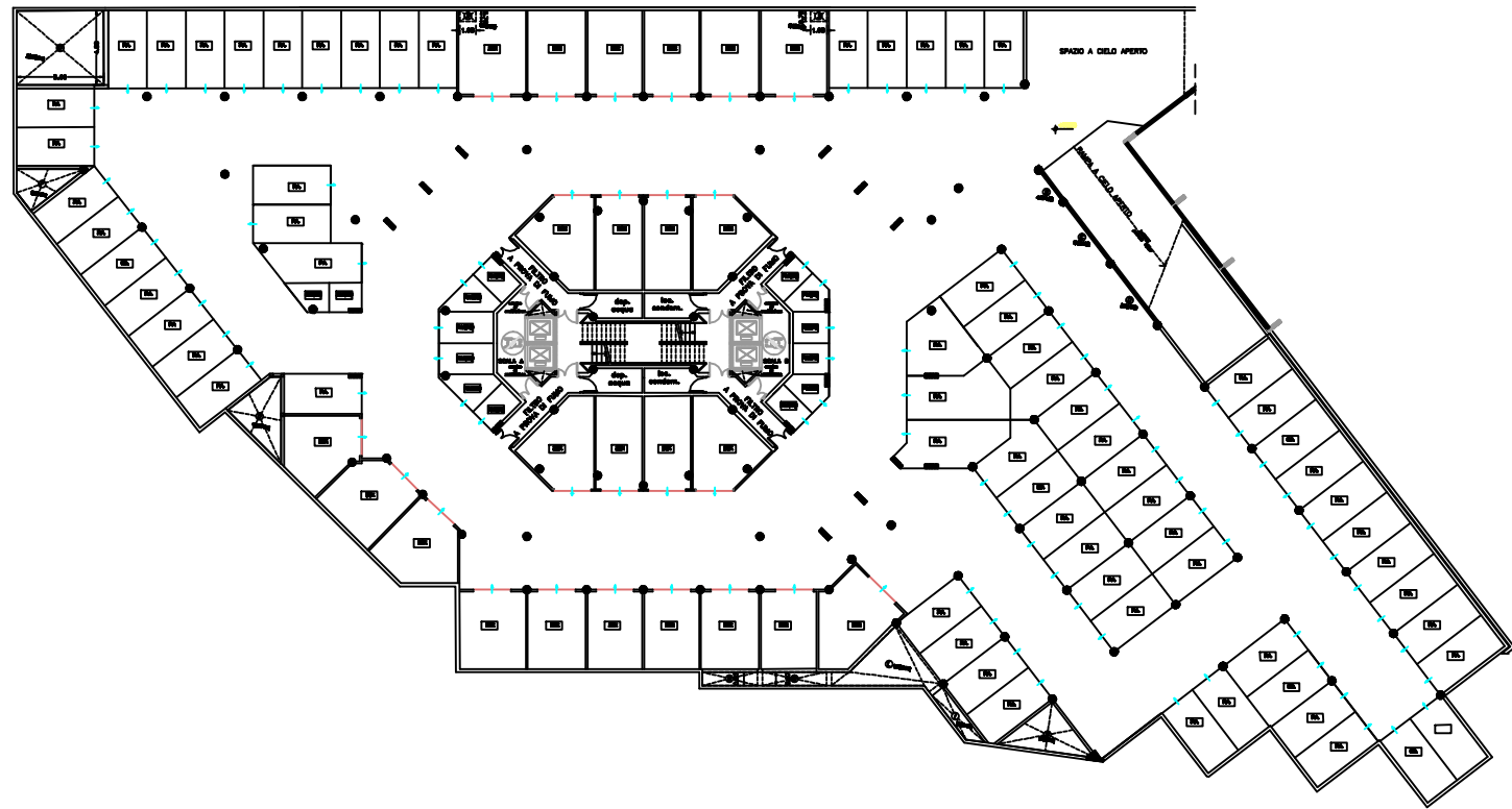
Piano autorimessa (2)
